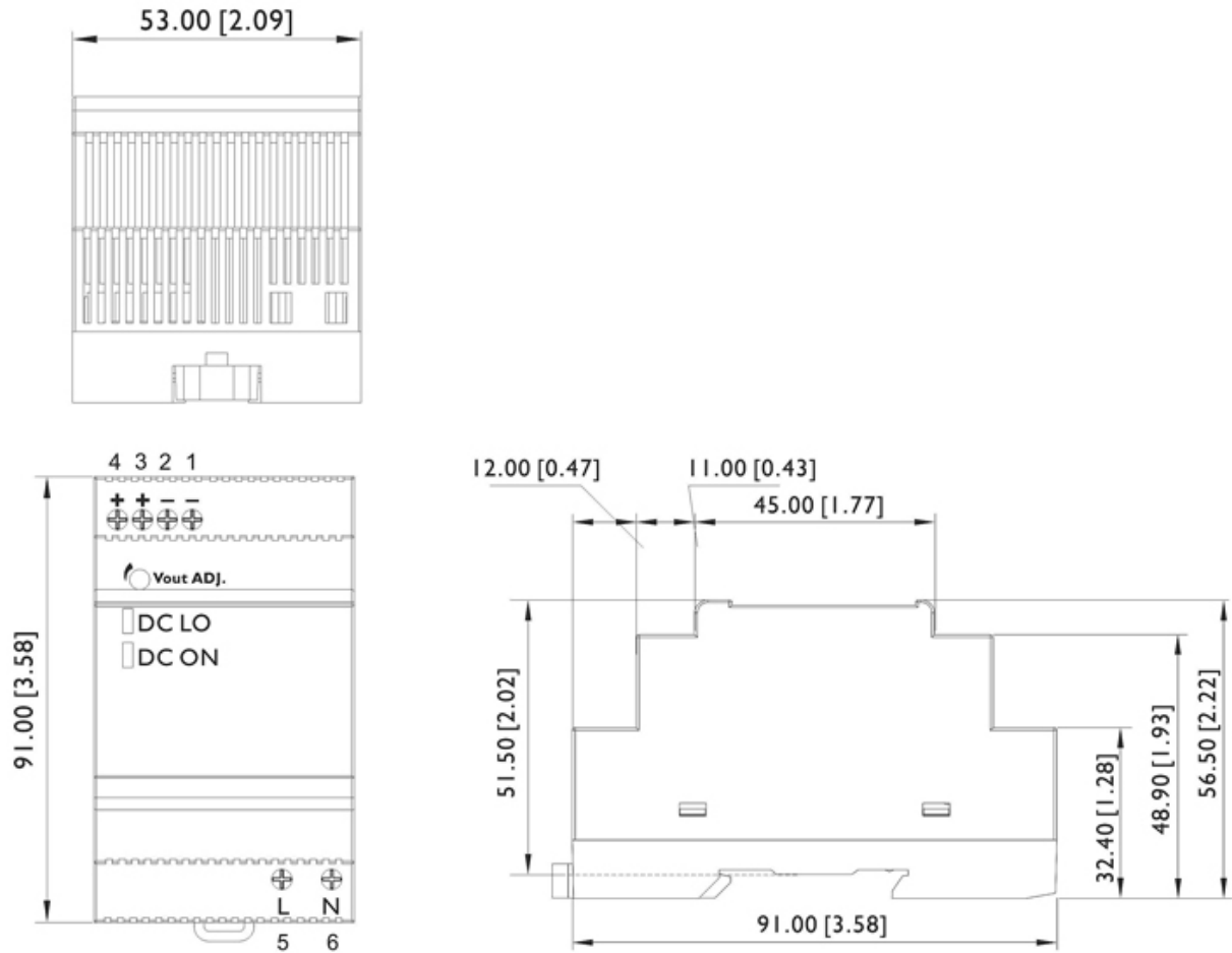
Abmessungen in mm [Inch]
