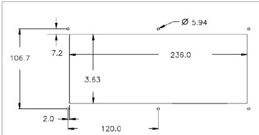
Schalttafelausschnitt (in mm)
