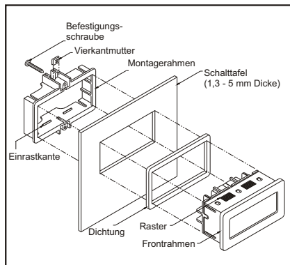
Bild 4.1: Montage
