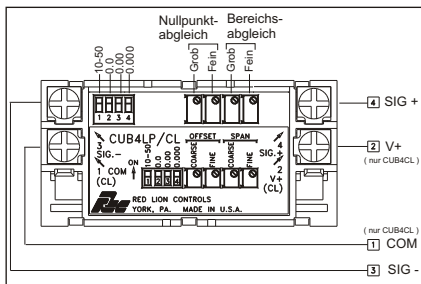
Bild 5.1: Anschlüsse
