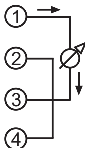
2-Draht Verbindung Aktiver Stromeingang.
