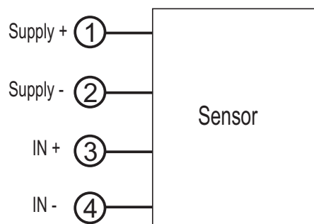
Aktiver Eingang von einem 4-Draht Sensor, versorgt über Hilfsversorgung.
