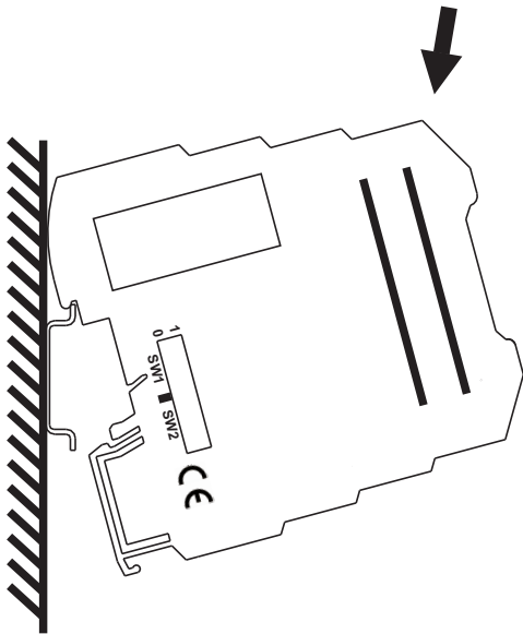
Montage des Moduls in der Schiene
