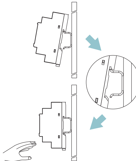
Bild 2: Montage
