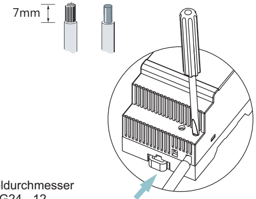
Bild: 3 Anschlussklemme
