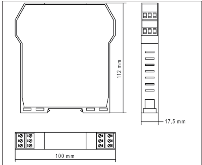
Abmessungen
