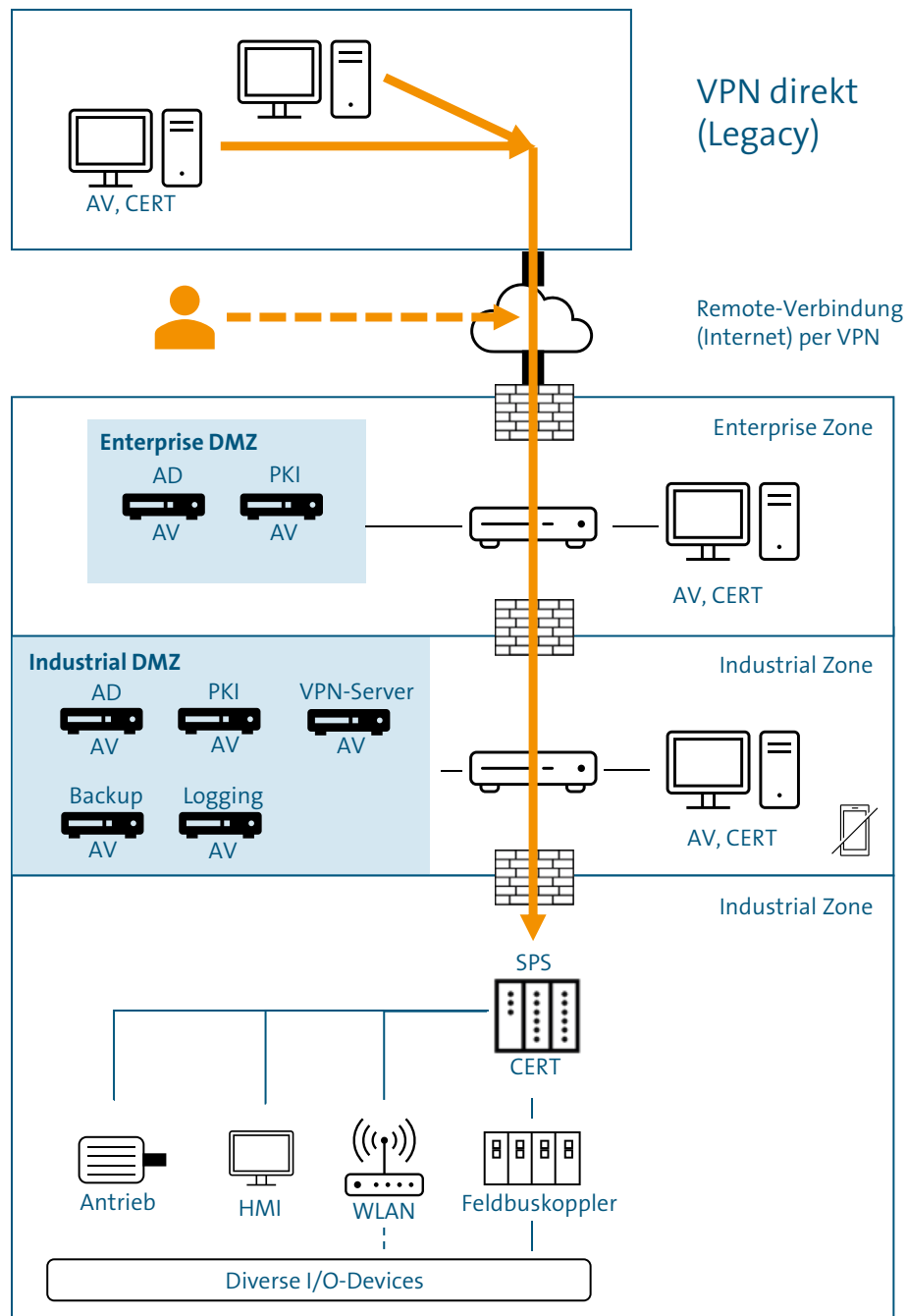
Abbildung 2 VPN direkt über Betreibernetzwerk
