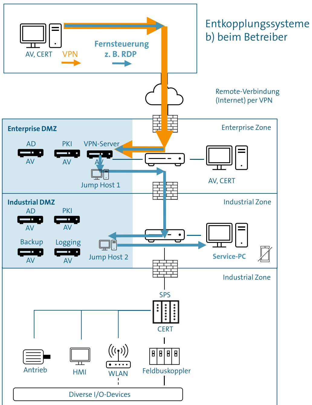
Abbildung 4 Entkopplungssysteme
