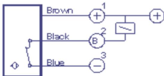
DC PNP, Schließer
