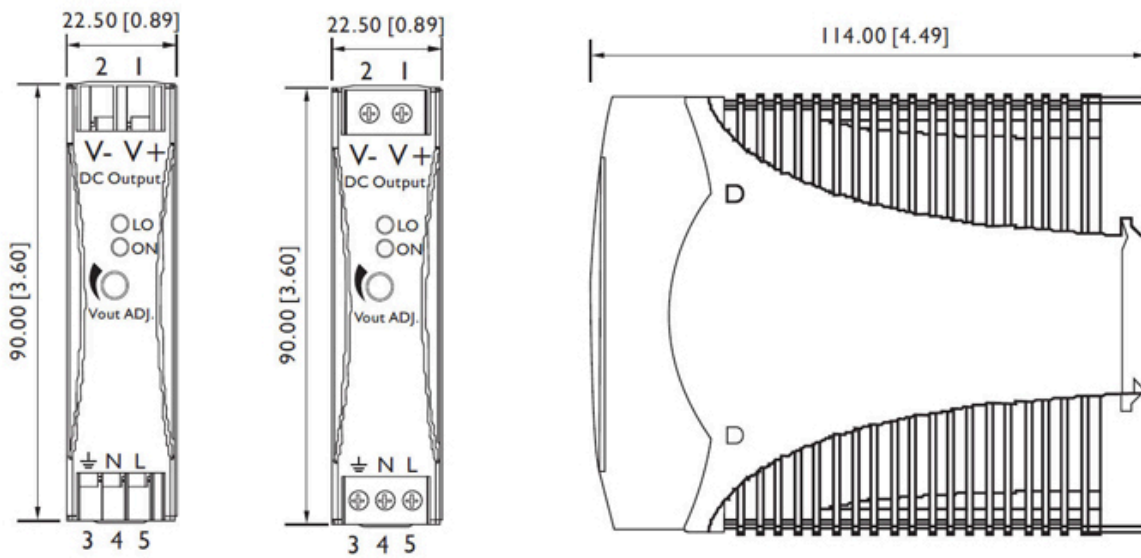
Abmessungen (mm/Inch)
