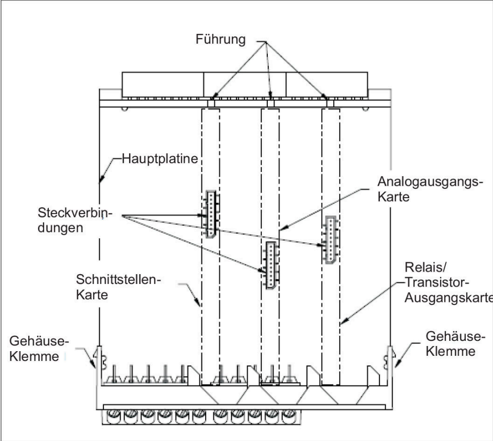
Mechanischer Aufbau
