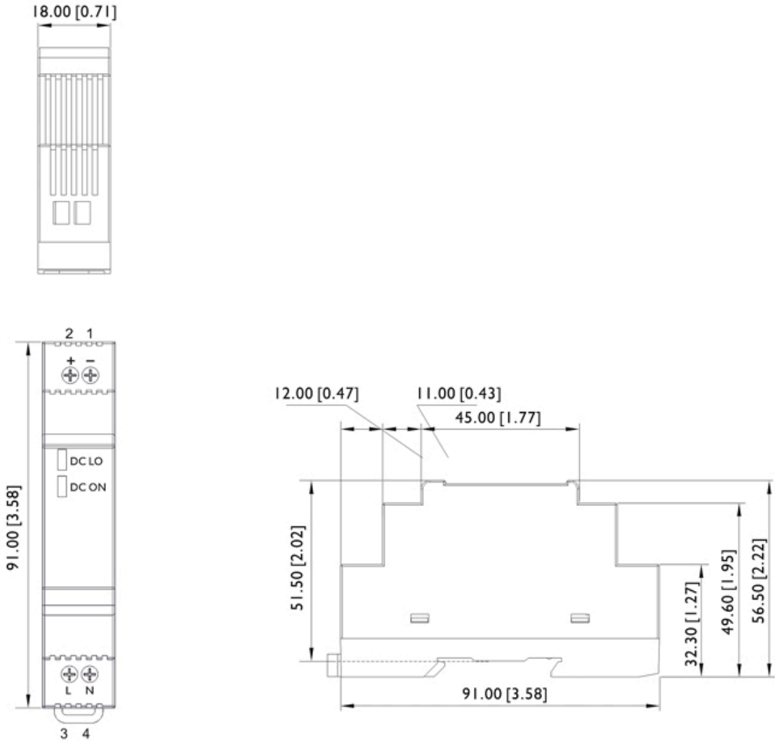
Abmessungen in mm [Inch]
