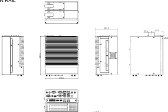
AVS-522 DIN RAIL
