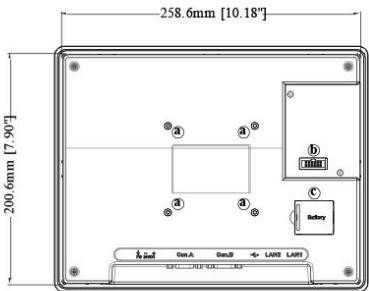
Rückansicht
