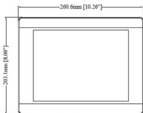
Frontansicht
