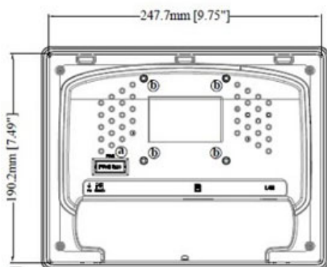
Rückansicht
