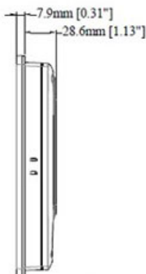
Seitenansicht
