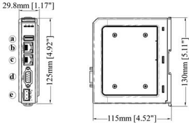
Frontansicht
