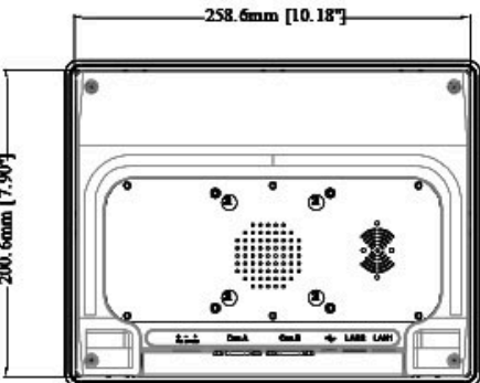
Rückansicht
