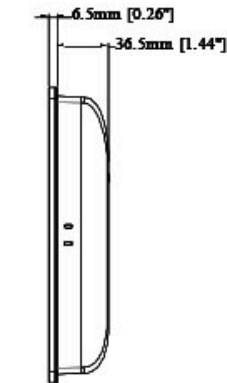
Seitenansicht
